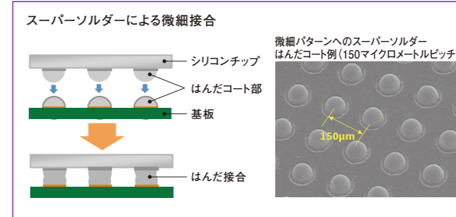
〈スーパー溶ダ〉 細かな部品の接合に優れた私たちの溶ダペースト「スーパー溶ダ」。微細接合部にスーパー溶ダを供給する当社の独自技術(はんだプリコート技術)は、今後ますます小型化する電子部品のはんだ接合に欠かせない技術として注目されています。
