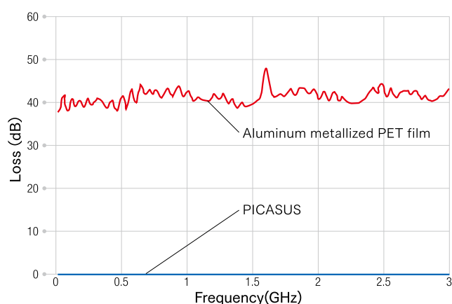
図 2：PICASUSの電波透過性
