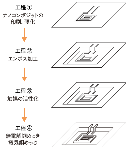
図 3：3次元配線の工程
