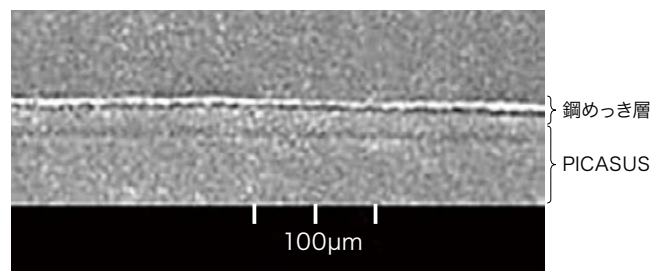
図 6：SEMによる銅めっき部分の断面観察
