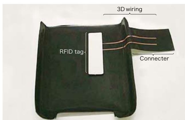
図8：RF-IDに接続した3次元配線
