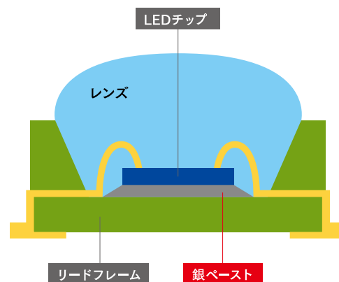
図2 LEDチップの構造
