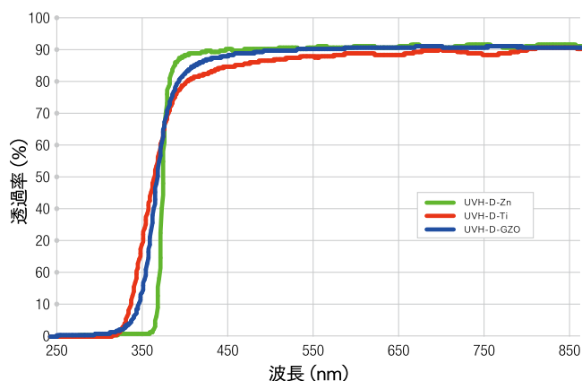
図1 分光透過率
